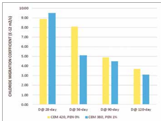
8. Attacco dei cloruri: coefficiente di migrazione ALFA
