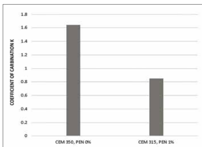
3. Resistenza alla carbonatazione: coefficient K di carbonatazione
